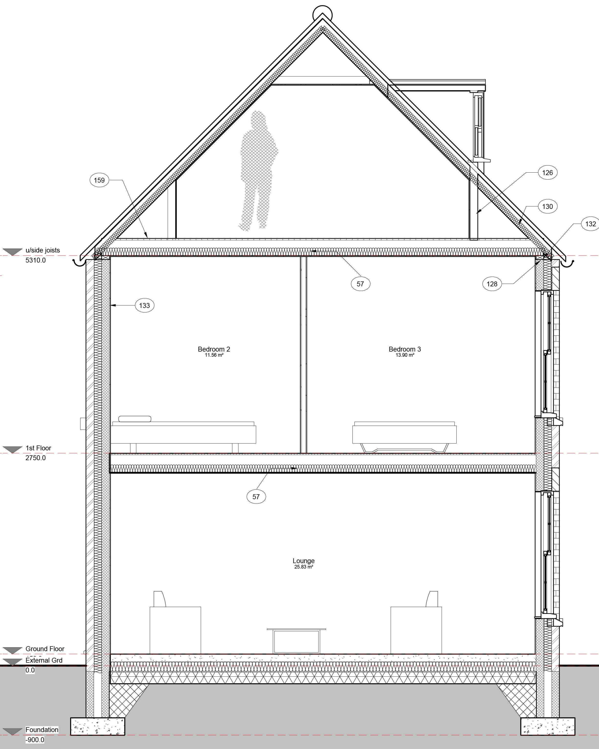
2 Main Section 1 : 25
