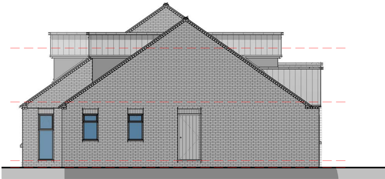
Elevation 04 - Left 1 : 100
