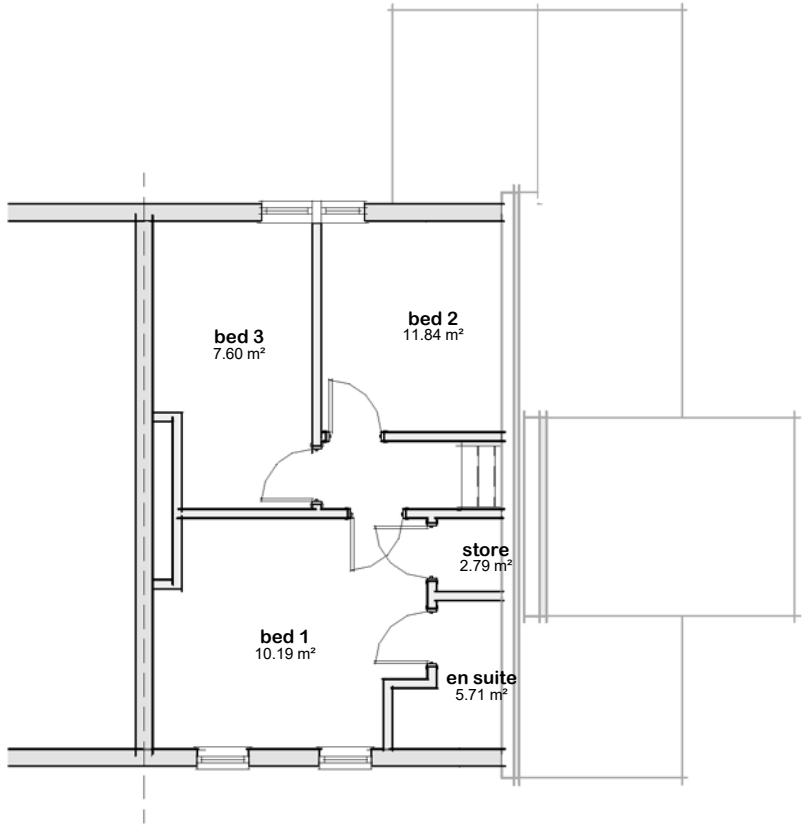
Plan 02 - First 1 : 100
