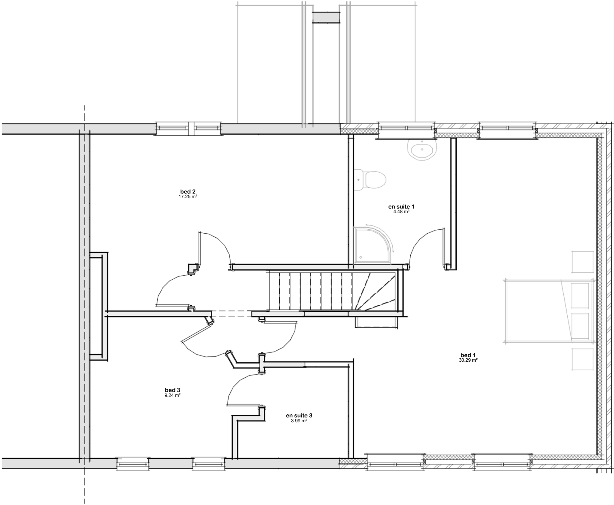
Plan 02 - First 1 : 50
