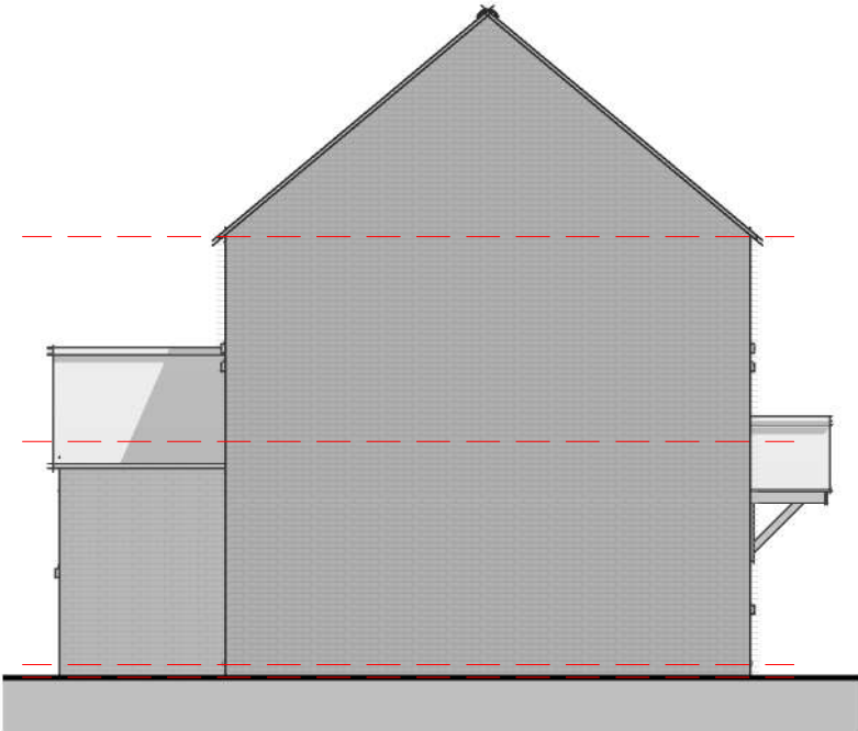
04 - Left Flank
