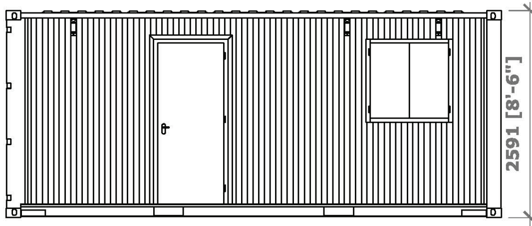
Elevation A
