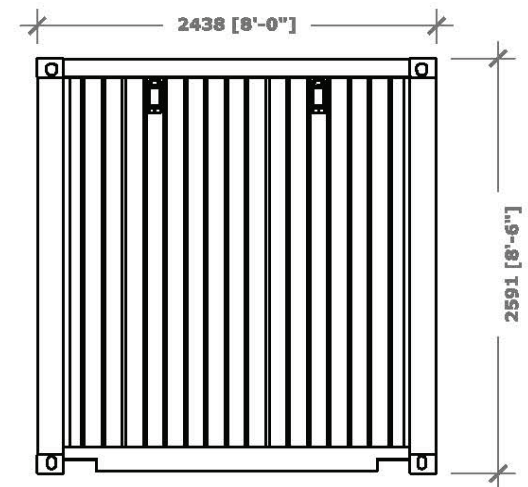
Elevation B
