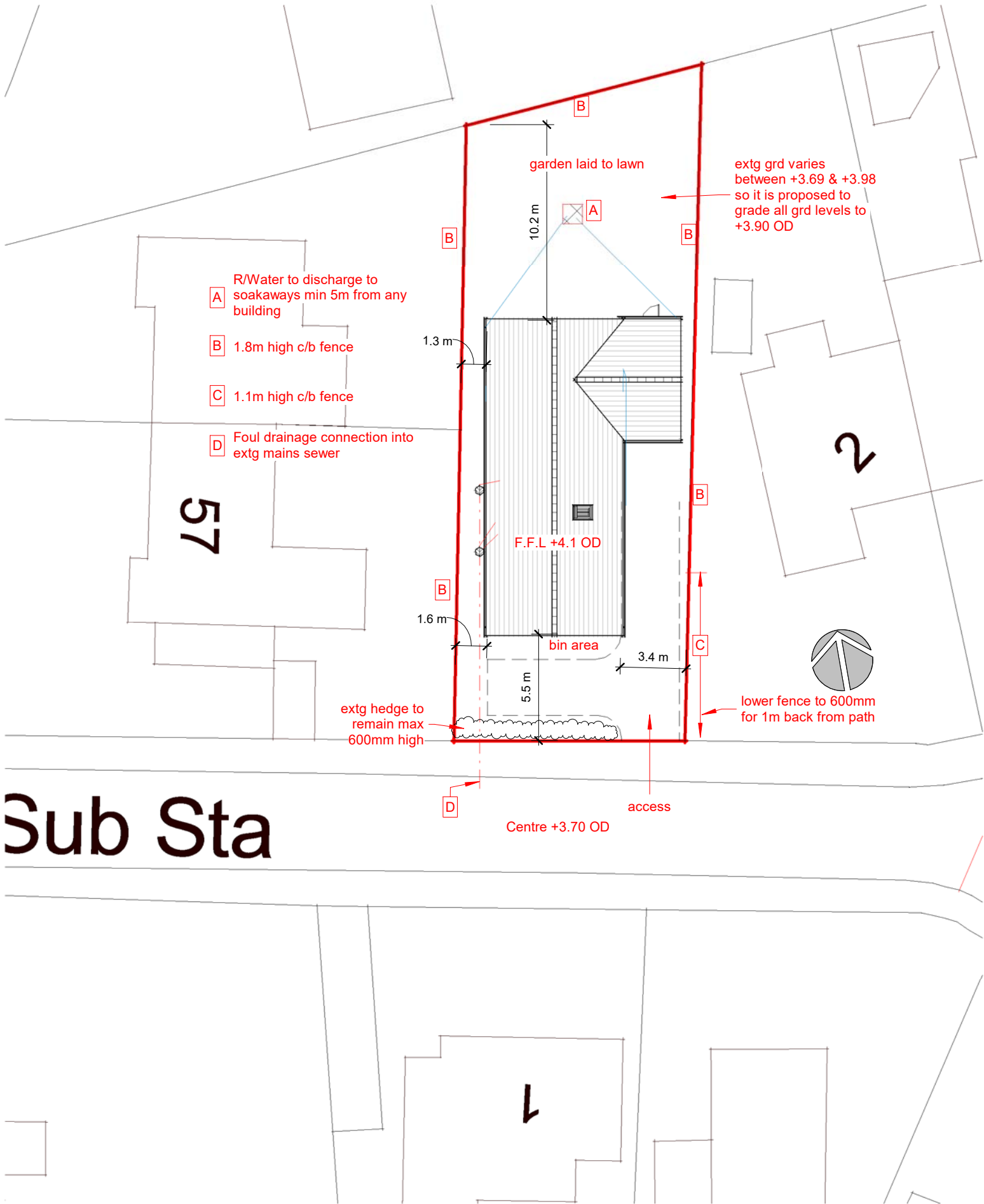
Site Block Plan 1 : 250
