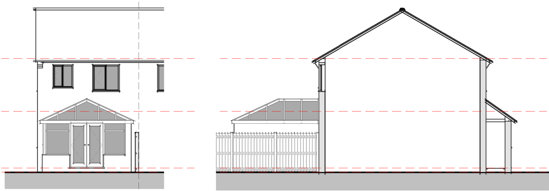
03-Rear 1 : 100
