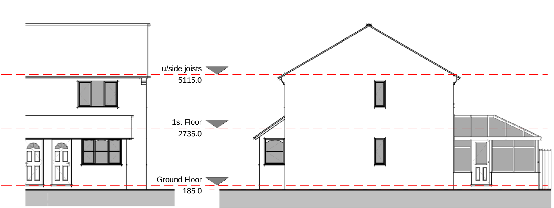
01-Front 1 : 100
