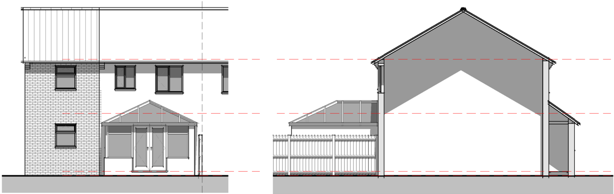
03-Rear 1 : 100
