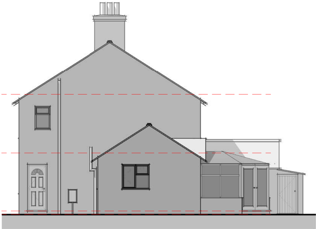
Elevation 02 - Right 1 : 100
