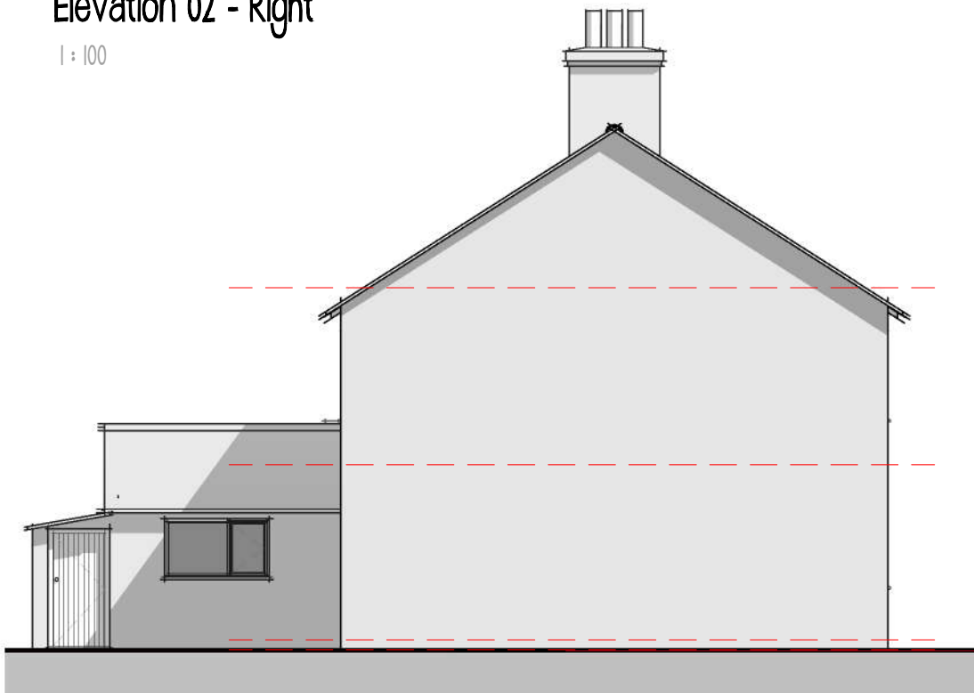
Elevation 04 - Left 1 : 100
