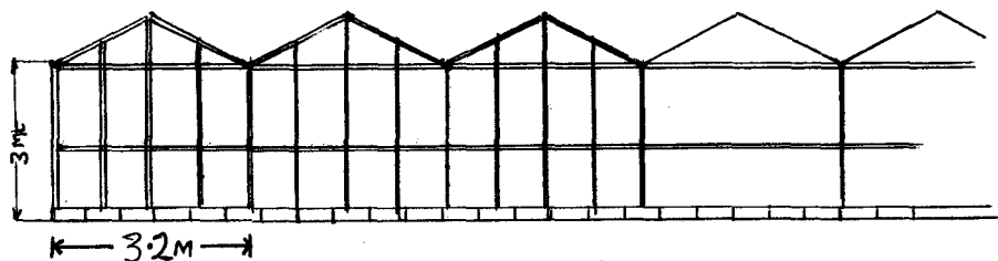
END ELEVATION
