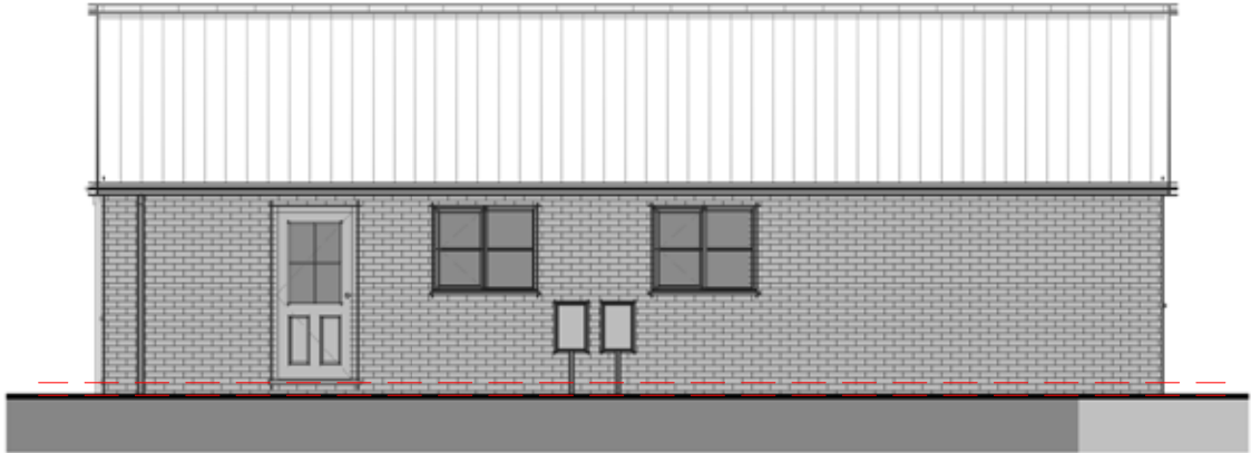
Elevation 04 - Left 1 : 100
