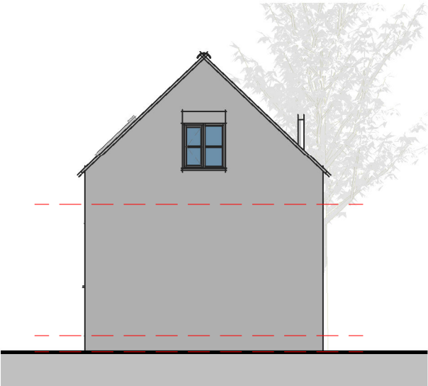
Elevation 04 - Left 1 : 100
