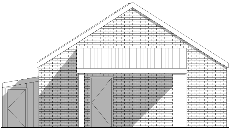
3 Existing Side B 1 : 100
