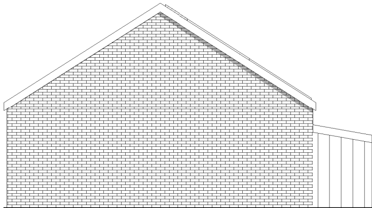
3 Existing Side A 1 : 100
