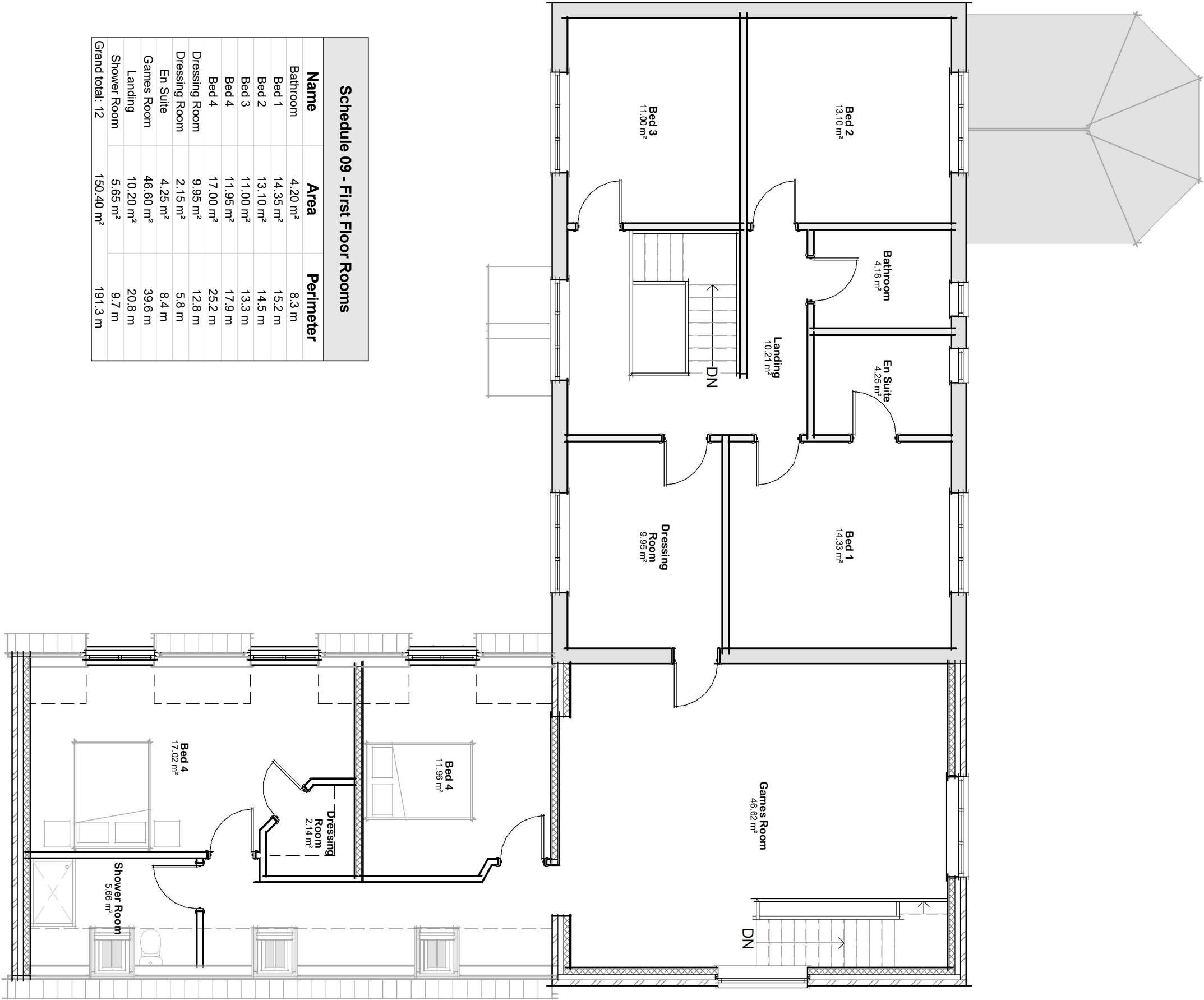
Plan 02 - First 1 : 75
