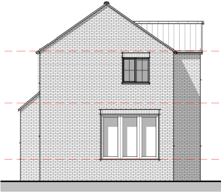
Elevation 02 - Right 1 : 100
