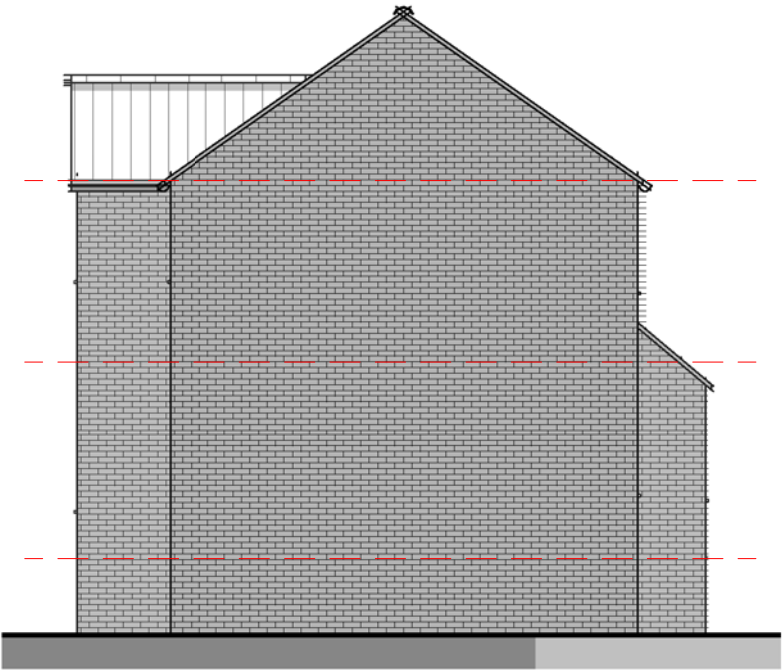
Elevation 04 - Left 1 : 100
