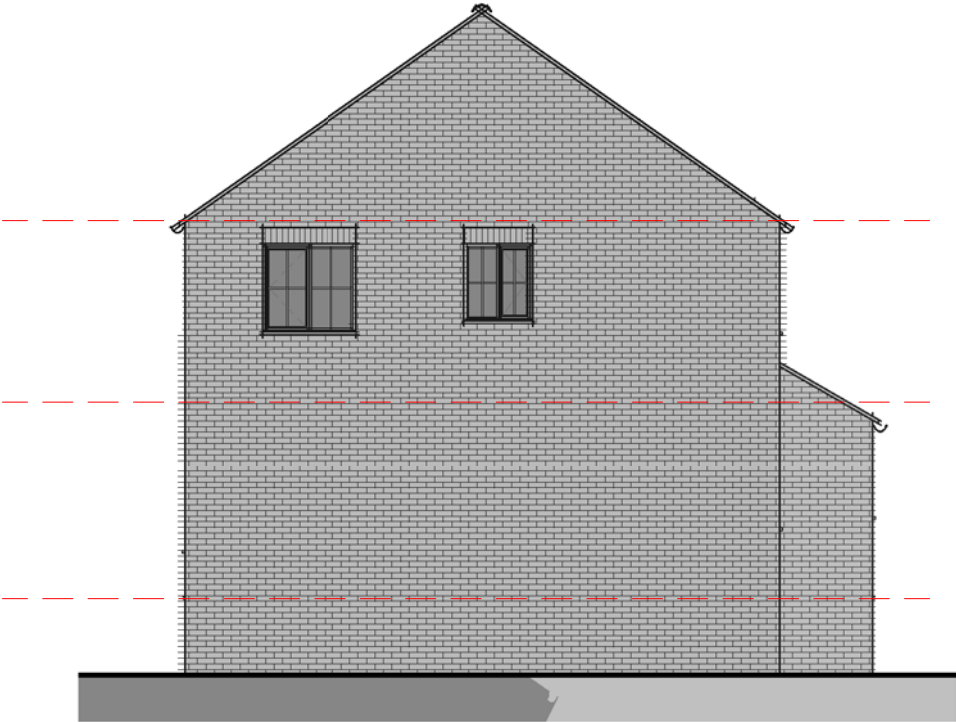
Elevation 04 - Left 1 : 100
