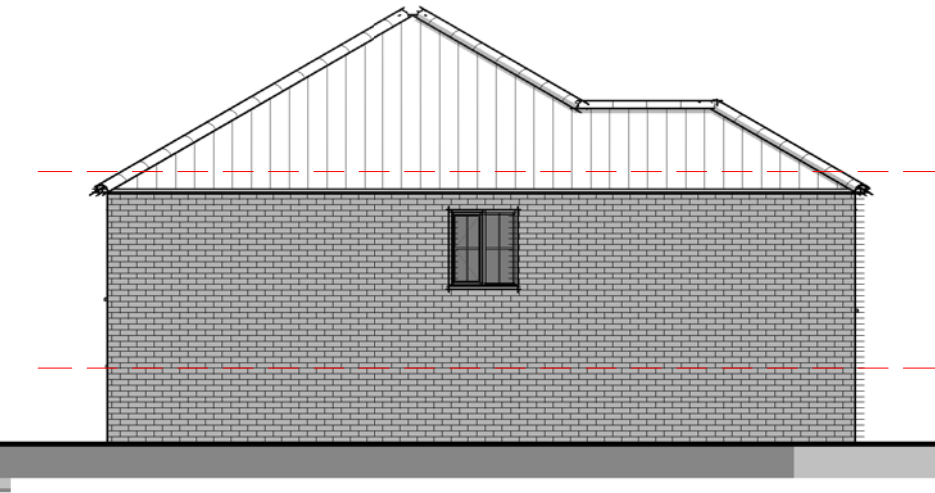
Elevation 04 - Left 1 : 100
