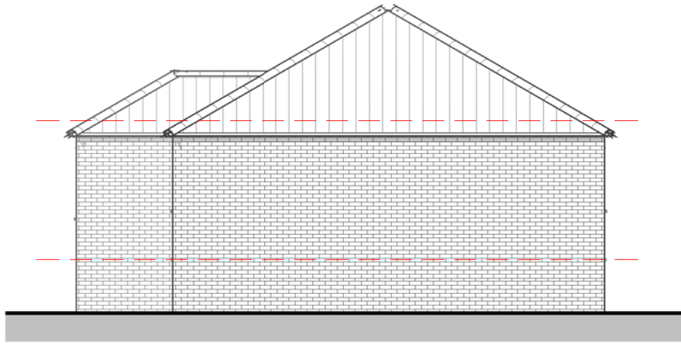
Elevation 02 - Right 1 : 100
