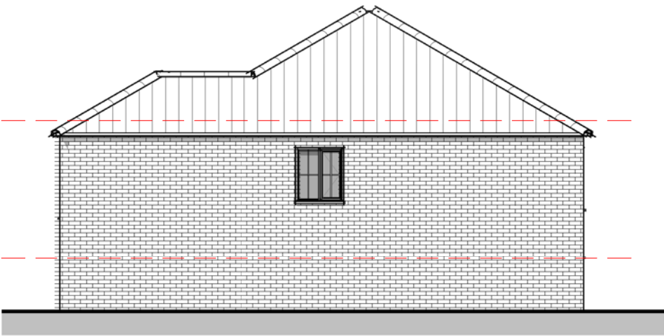
Elevation 02 - Right 1 : 100
