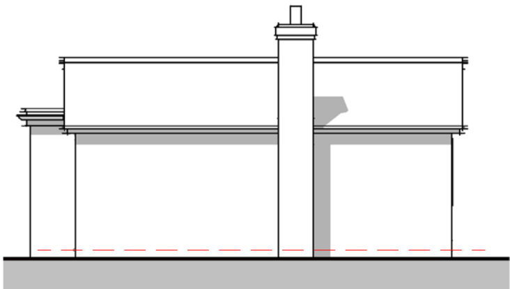
Elevation 04 - Left 1 : 100
