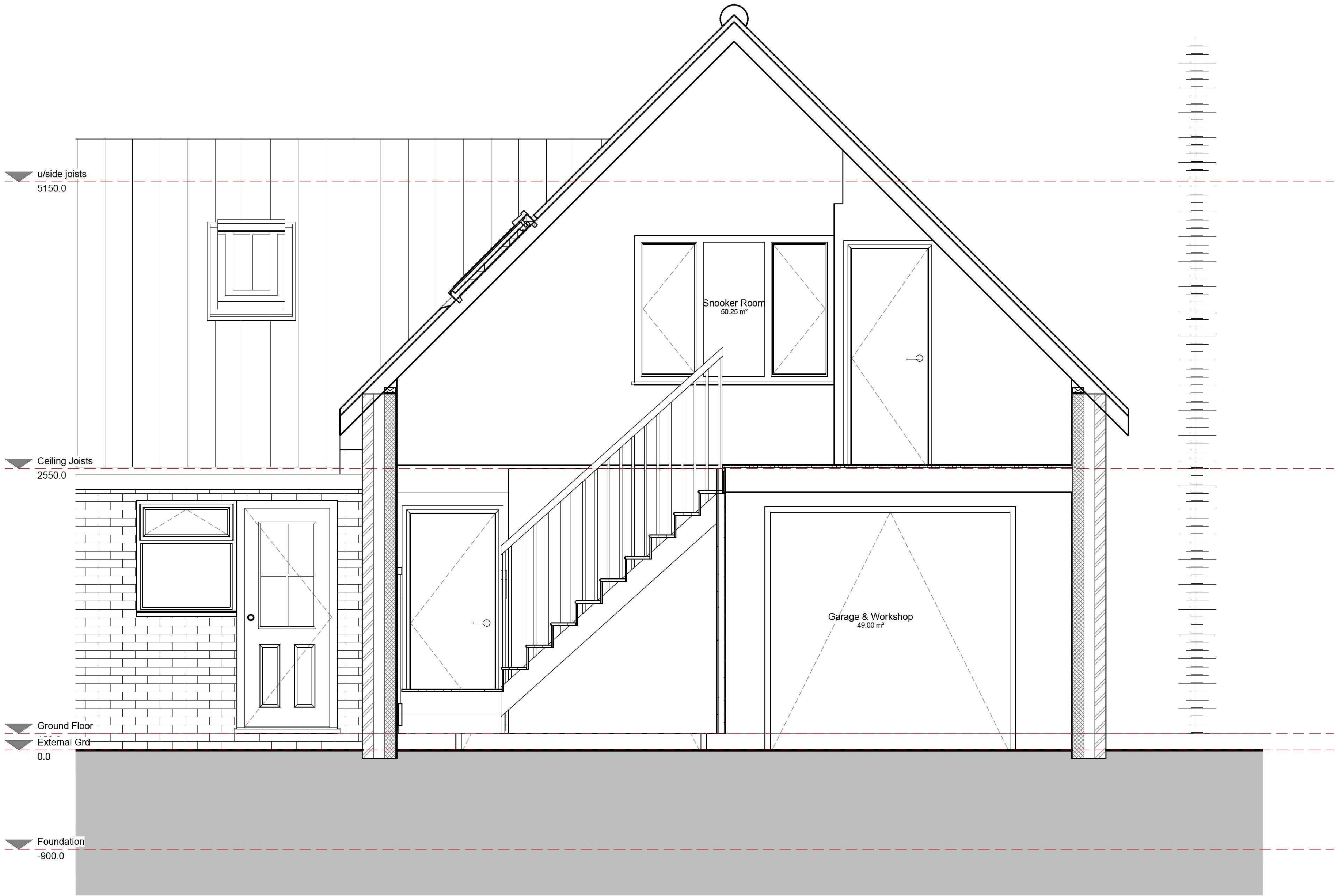
1 Garage Section 1 : 25
