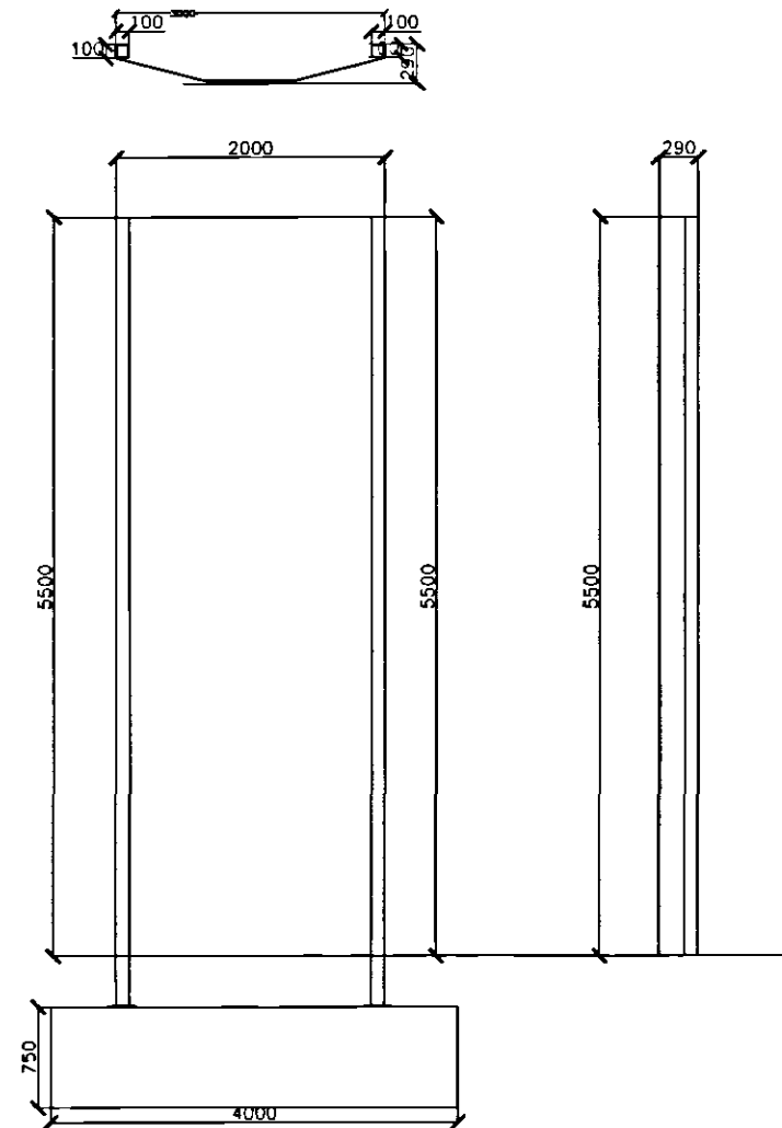
Type 2A - Tatum Signage (adj to NFU corner) 1:50
