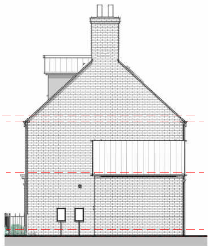
Elevation 02 - Right 1 : 100
