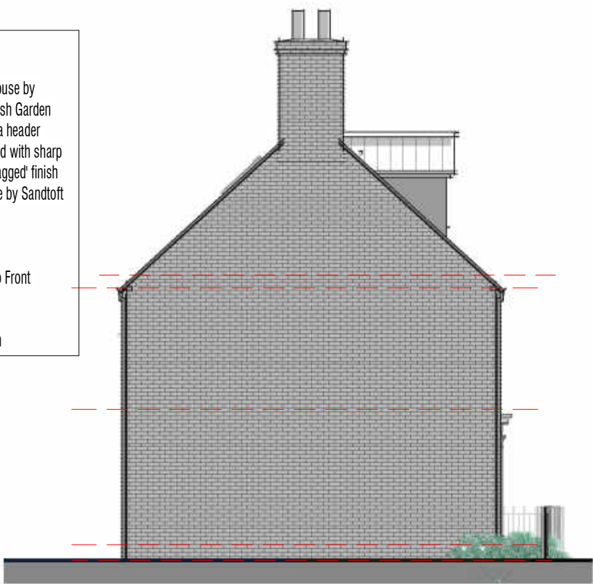
Elevation 04 - Left 1 : 100
