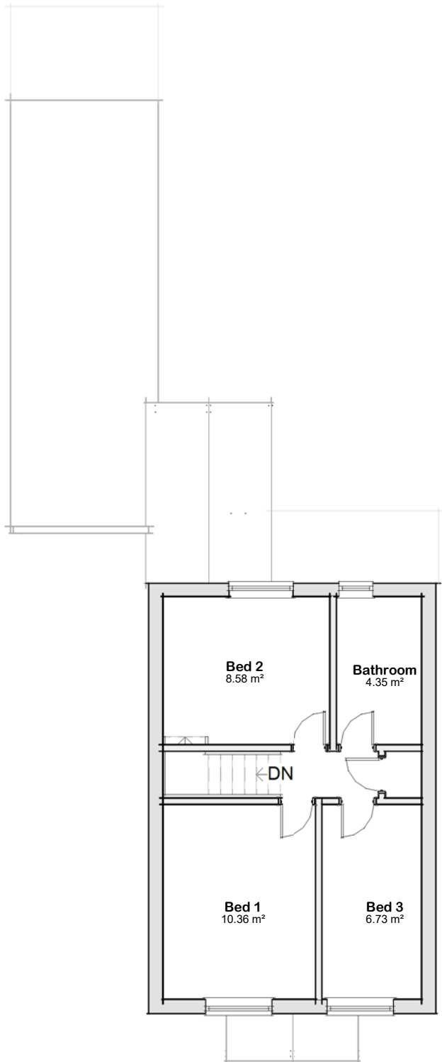
Plan 02 - First 1 : 100
