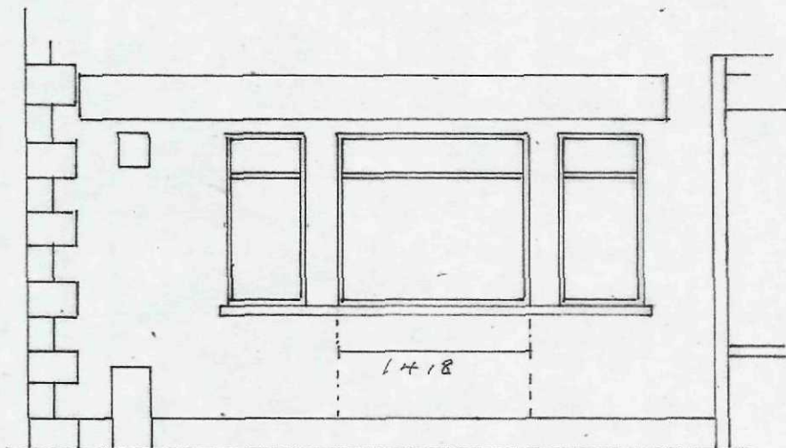
Existing 1:100
