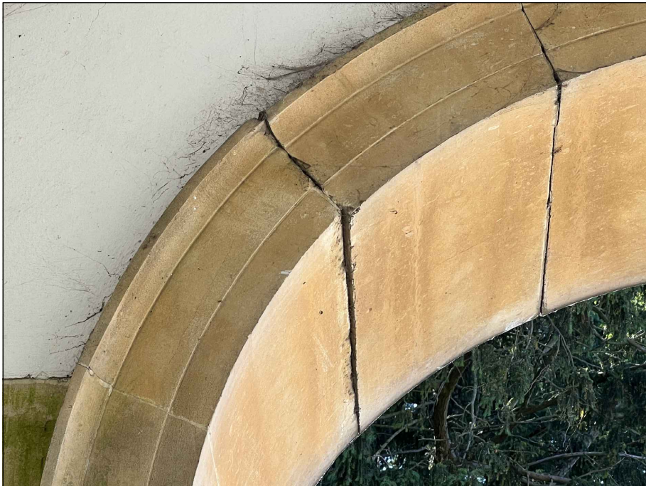
Arch 5 - Slipped voussoirs
