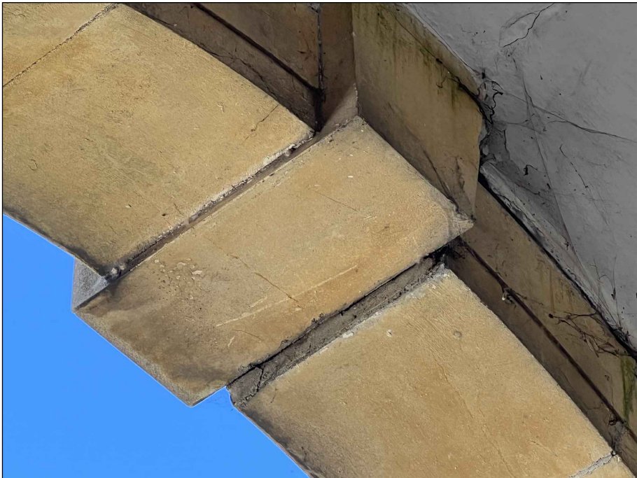
Arch 2 slipped voussoirs
