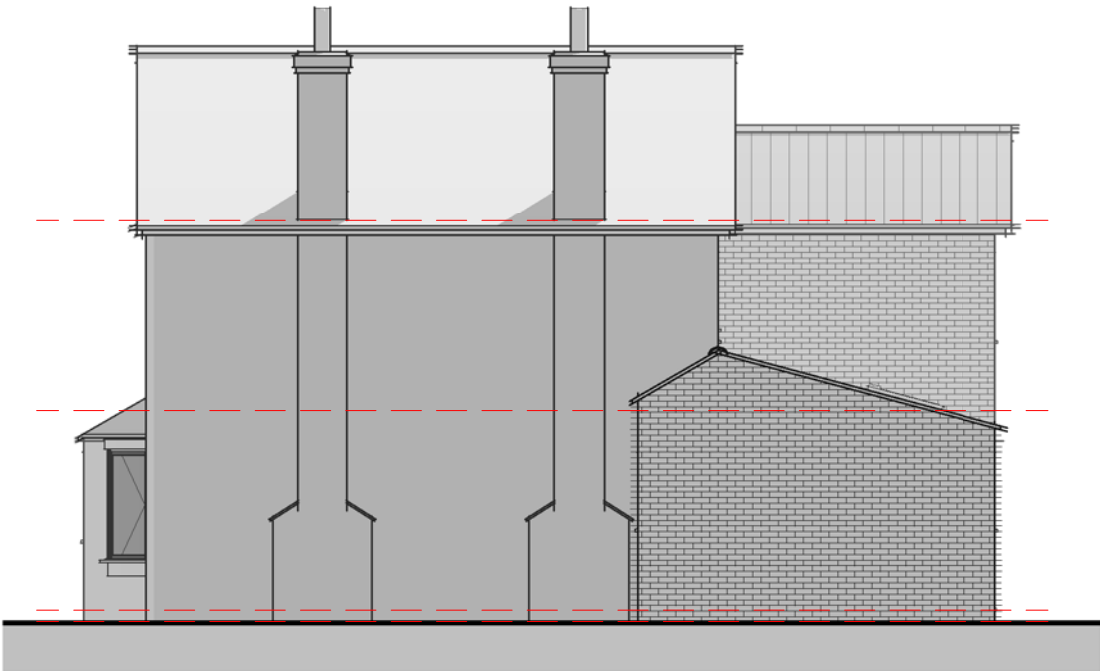
Elevation 02 - Right 1 : 100
