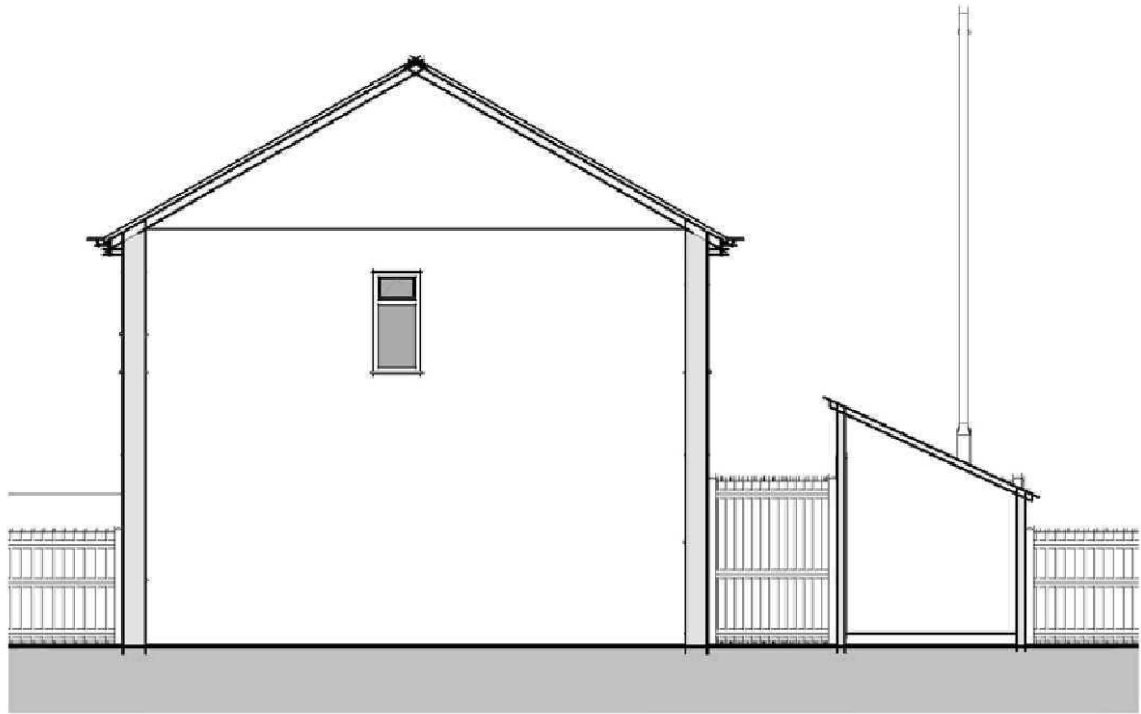
02 - Right Flank 1 : 100
