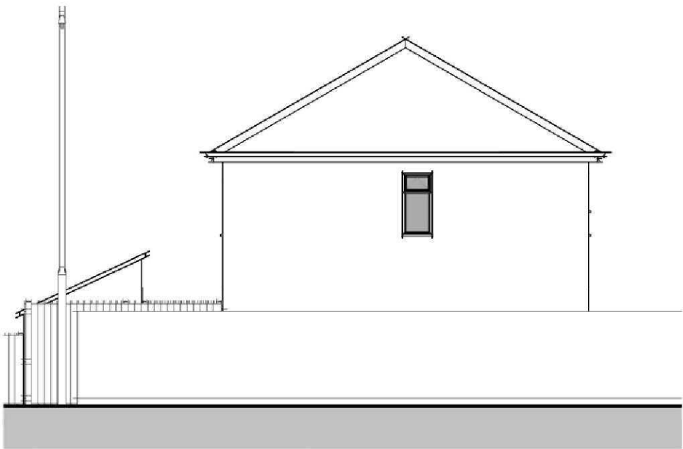
04 - Left Flank 1 : 100
