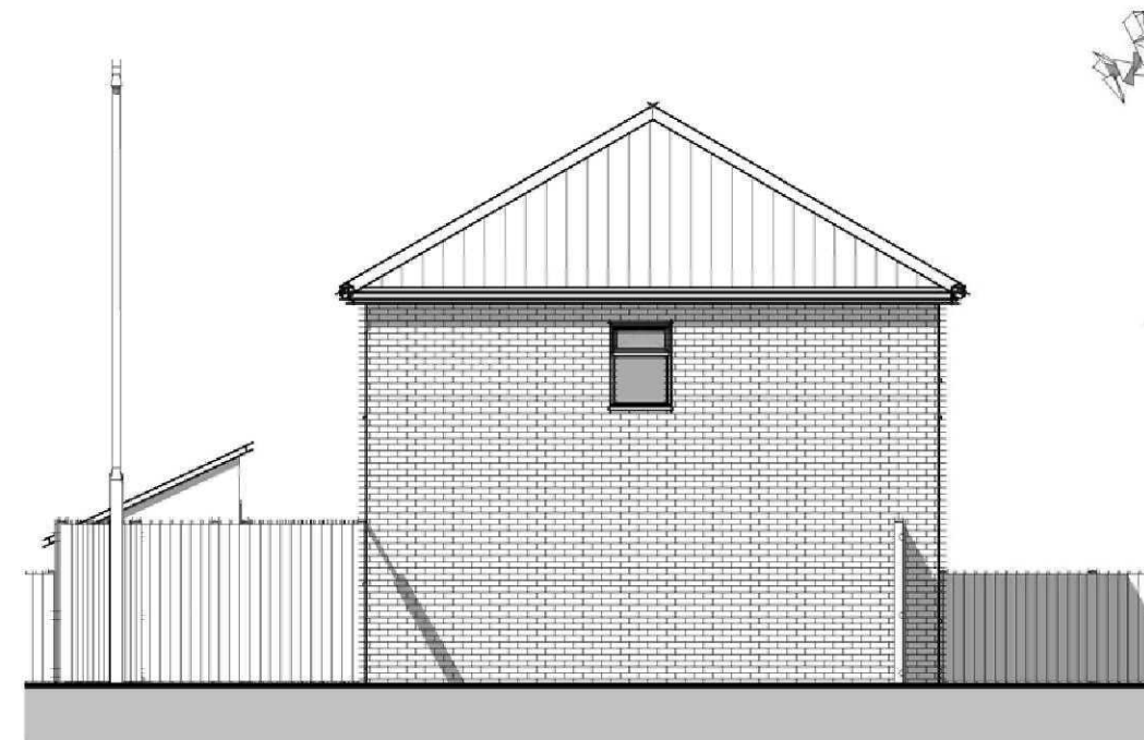
04 - Left Flank 1 : 100
