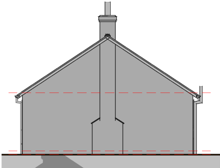
Elevation 02 - Right 1 : 100
