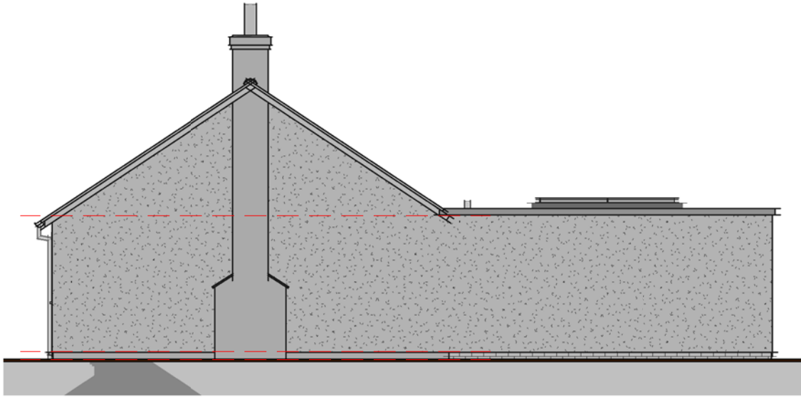
Elevation 02 - Right 1 : 100
