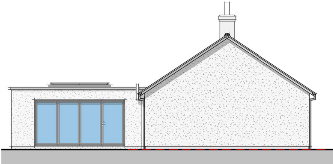
Elevation 04 - Left 1 : 100
