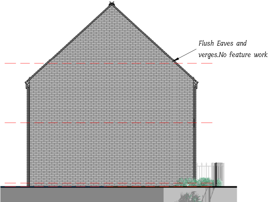
Elevation 02 - Right 1 : 100
