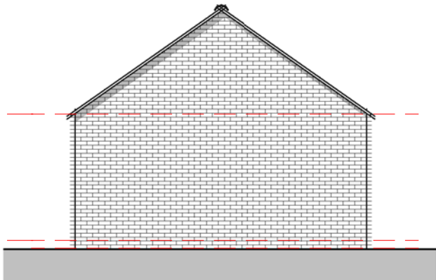
Elevation 02 - Right 1 : 100
