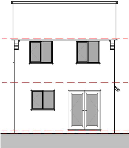
03 - Rear 1 : 100
