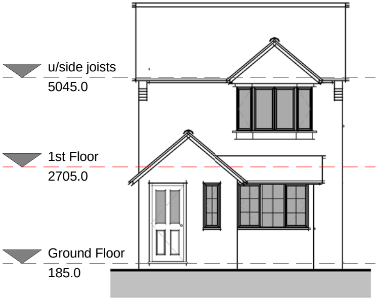
01 - Front 1 : 100
