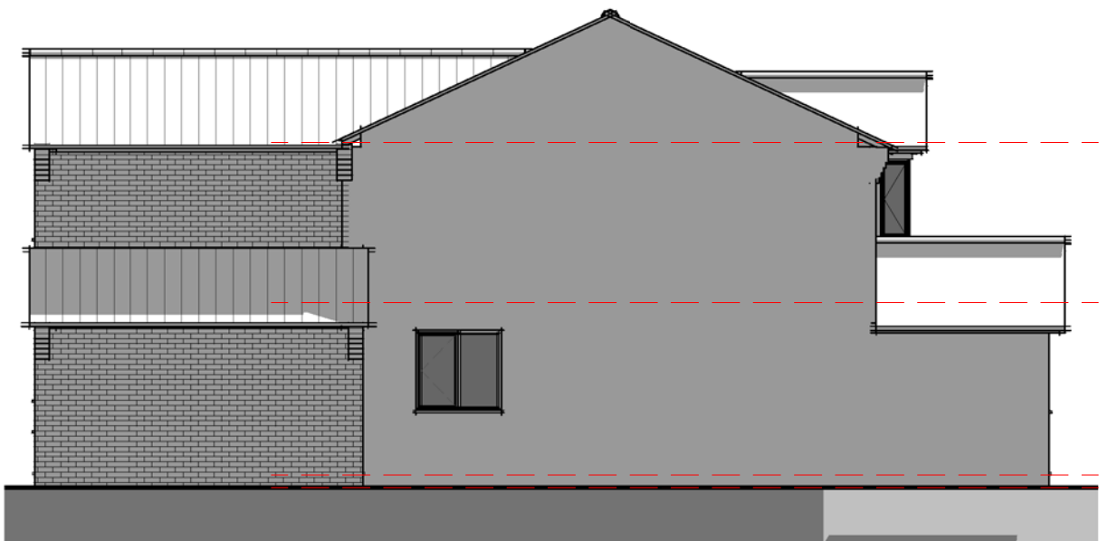
04 - Left Flank 1 : 100
