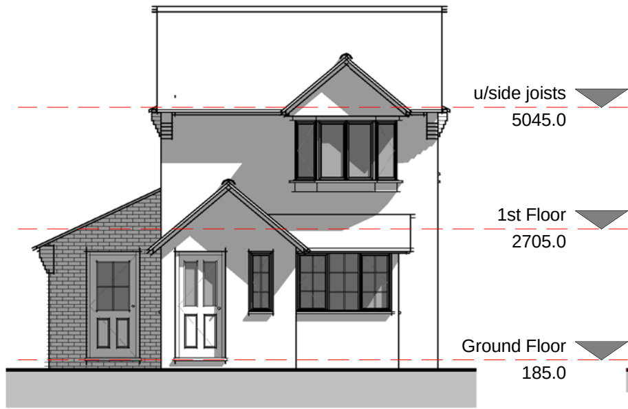
01 - Front 1 : 100
