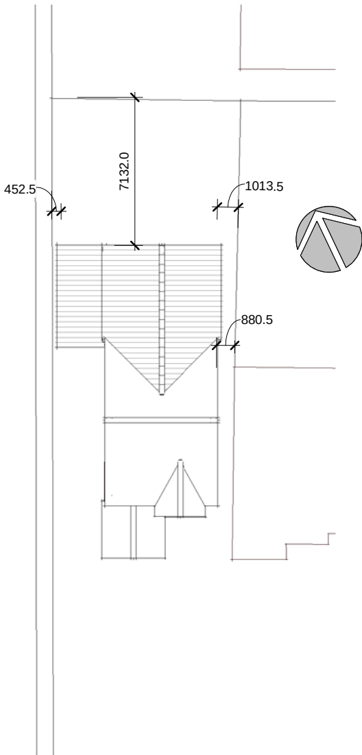
Site Block Plan 1 : 250
