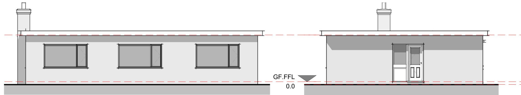
Elevation 02 - Right 1 : 100
