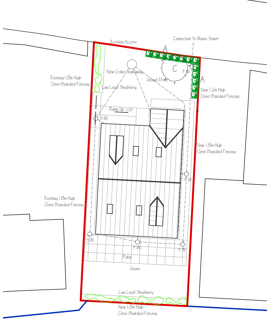
SITE PLAN 1:200
