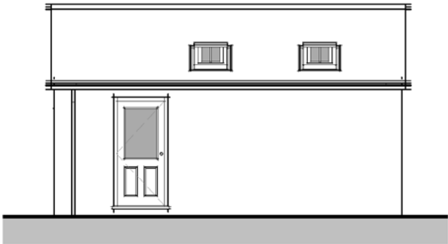
02 - Right Flank 1 : 100
