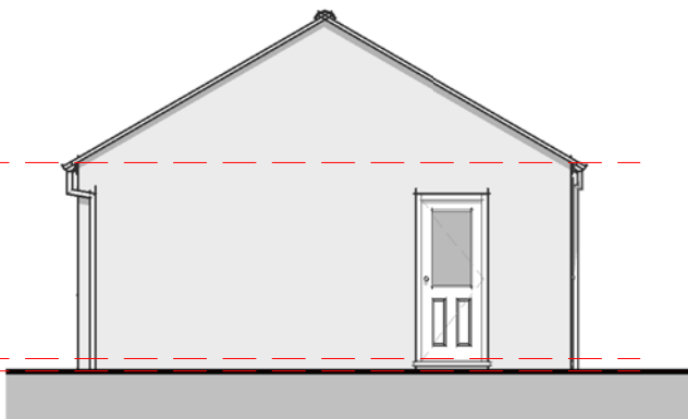
Elevation 02 - Right 1 : 100
