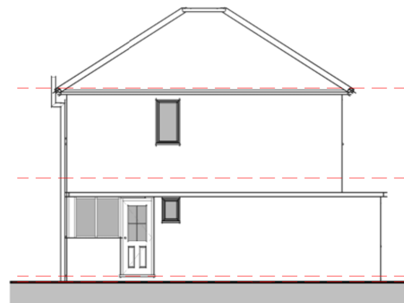
Elevation 04 - Left 1 : 100
