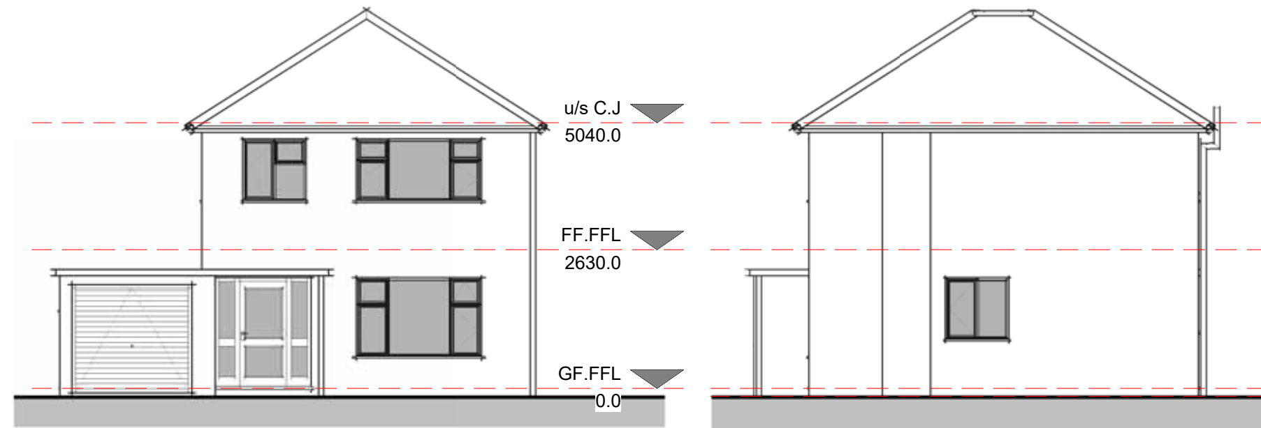
Elevation 02 - Right
