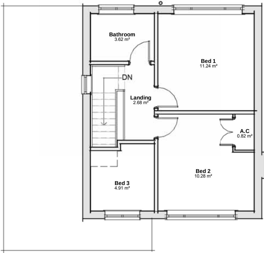
Plan 02 - First 1 : 75
