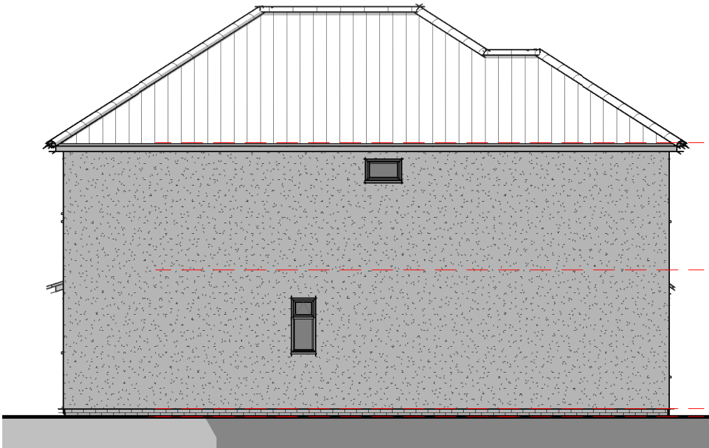
Elevation 04 - Left 1 : 100
