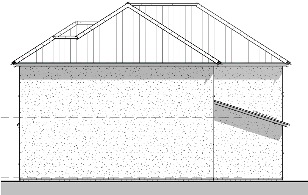
Elevation 02 - Right 1 : 100
