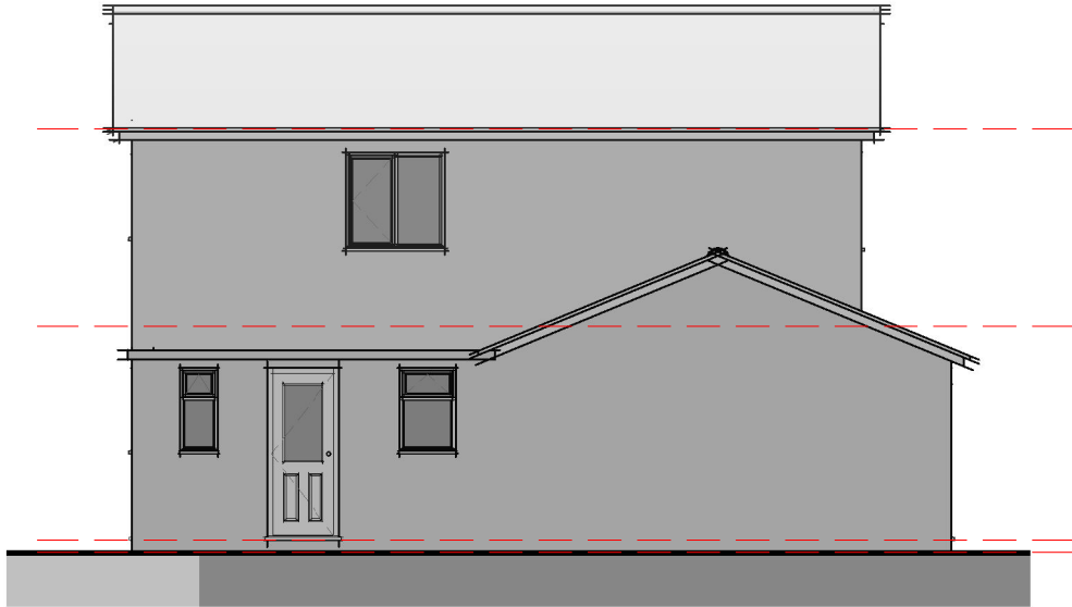
Elevation 04 - Left 1 : 100
