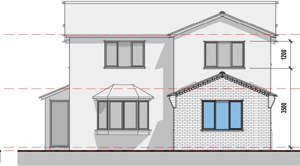
Elevation 02 - Right 1 : 100
