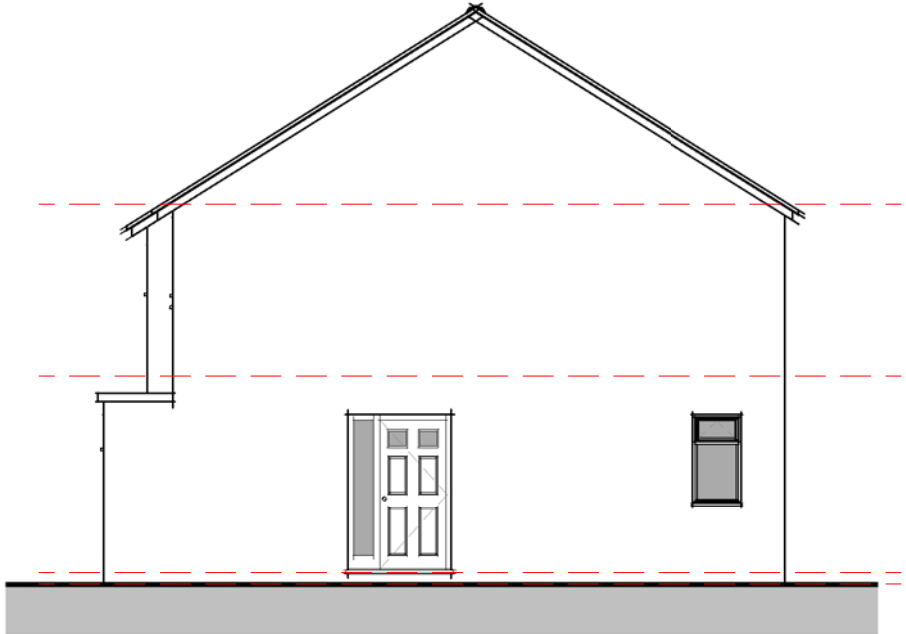
Elevation 04 - Left 1 : 100
