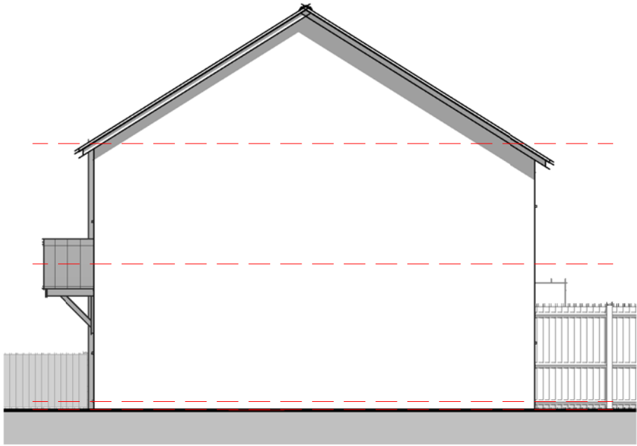
Elevation 02 - Right 1 : 100
