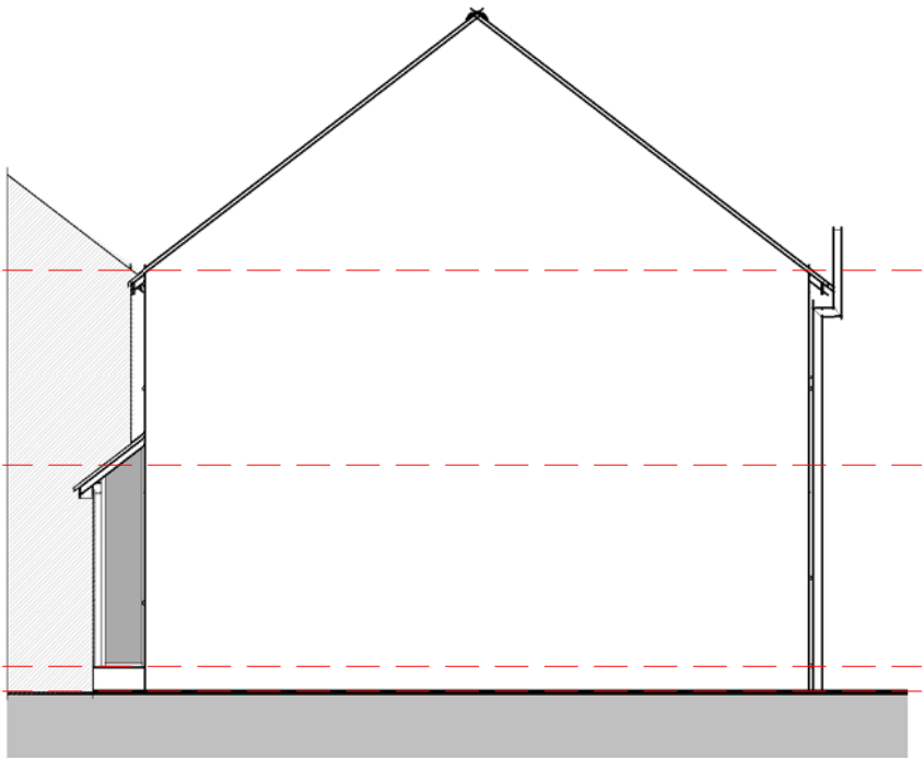
02 - Right Flank 1 : 100
