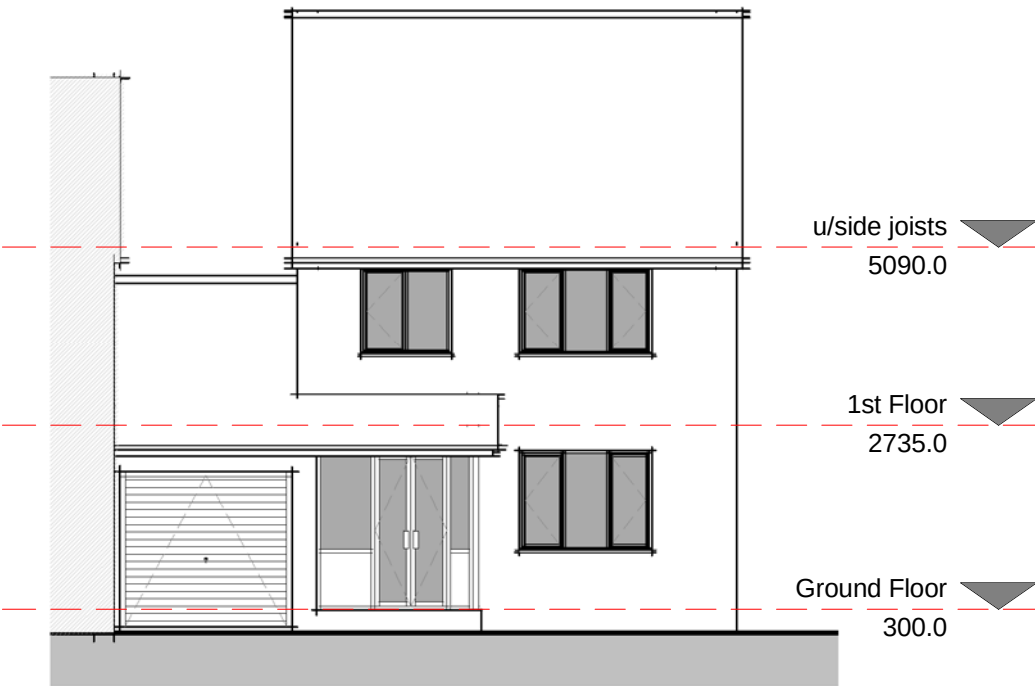
01 - Front 1 : 100
