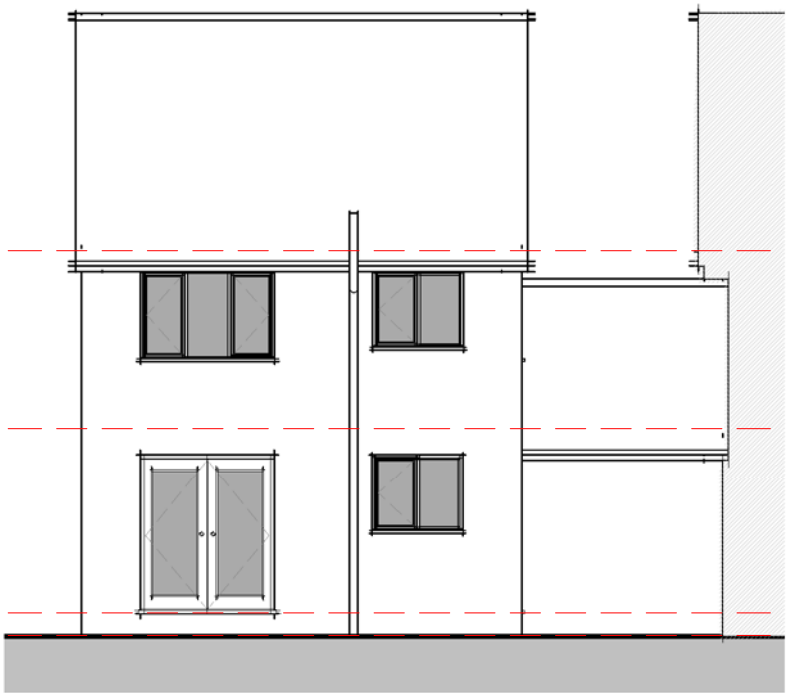
03 - Rear 1 : 100
