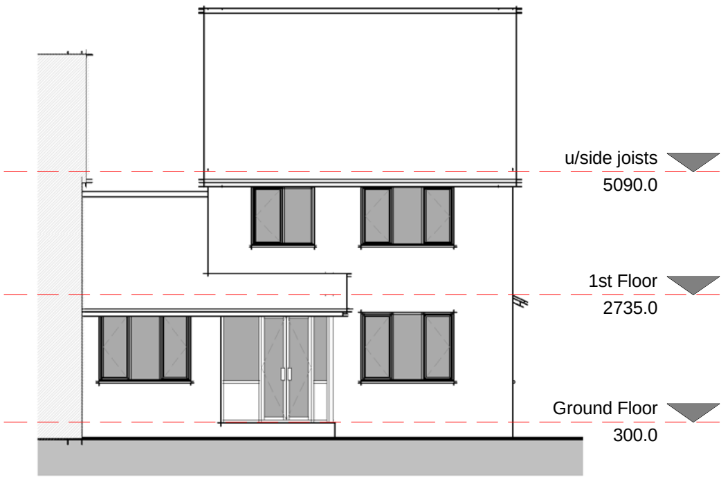
01 - Front 1 : 100
